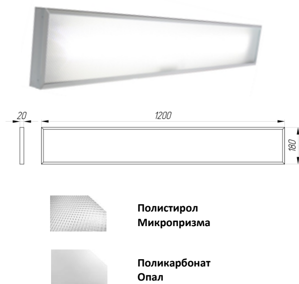
Рисунок 1 – Внешний вид.
