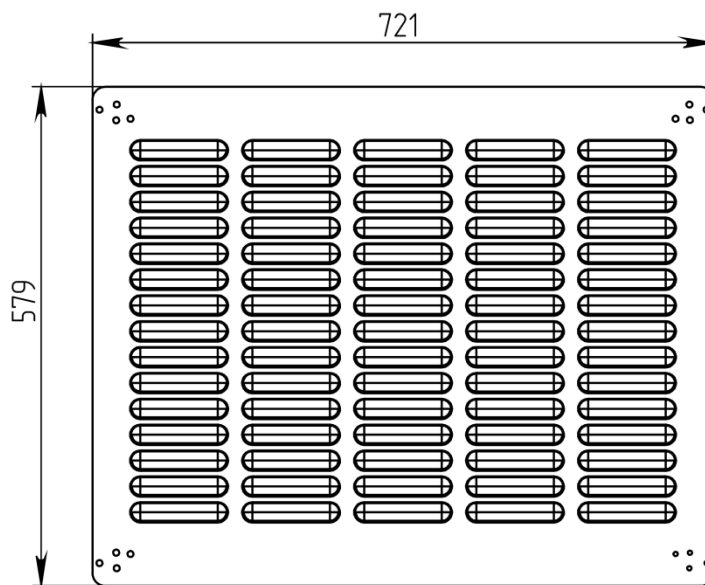
Рисунок 2 – Габаритный чертеж.
