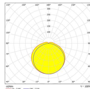
Рисунок 3 – Светораспределение светильника Geniled Лайнер-X 11W 5000К.
