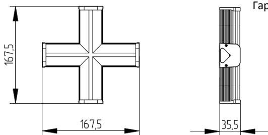
Рисунок 2 – Габаритные размеры светильника Geniled Лайнер-X 11W 5000К.
