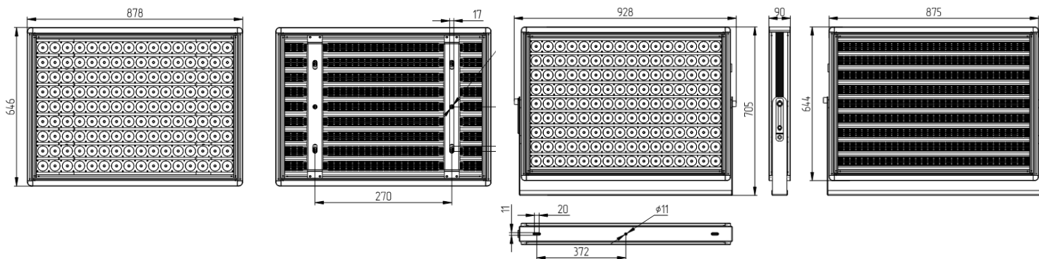
Рис.1 Габаритный чертеж прожектора Geniled Solar 1500 с креплением на два кронштейна.
