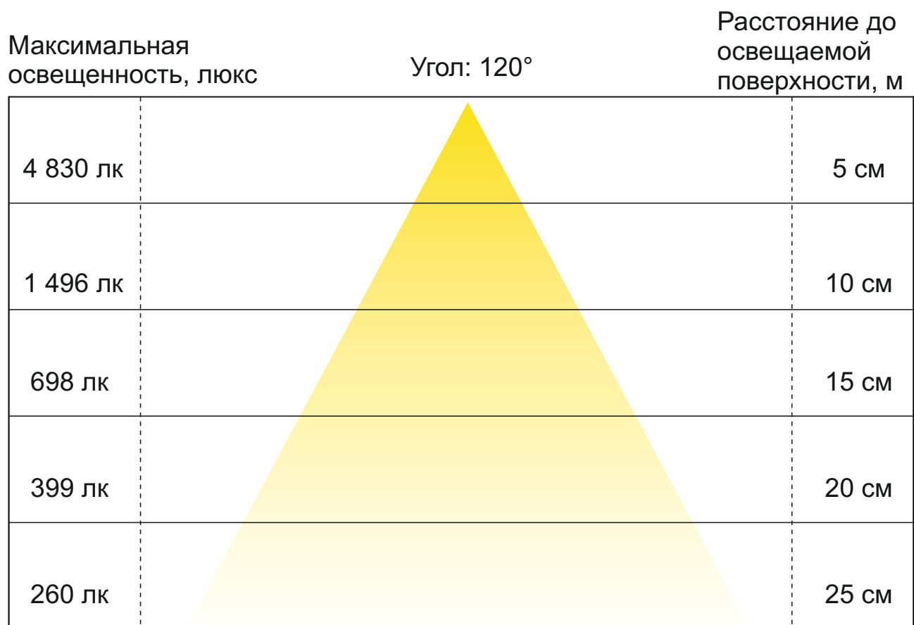
Светодиодный модуль Geniled GL-4SMD5050, 80 Лм, 1 Вт
